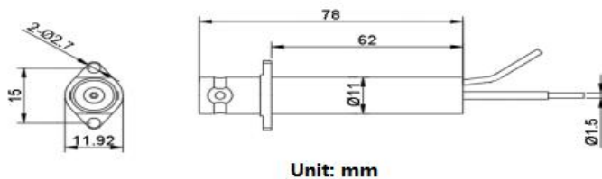
(CSD050, CSD100 机械规格)
